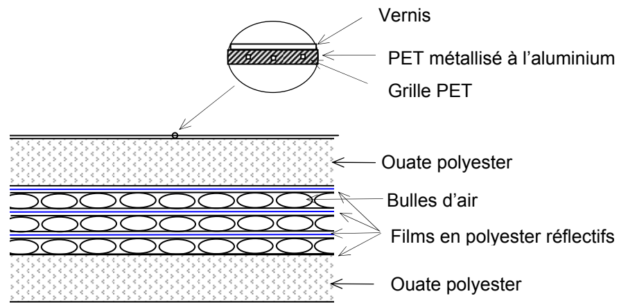
Figure 1 : schéma en coupe du produit
