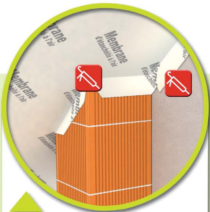
Raccordement sur boisseaux isolés
