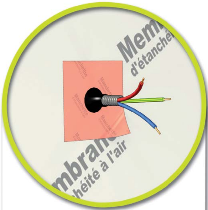
Traversée de membrane par une gaine
