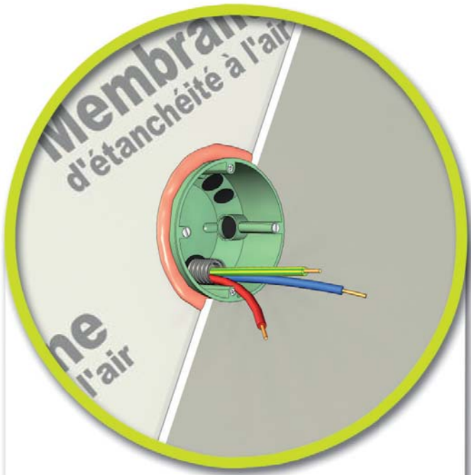
Pose d'un boîtier électrique plein
