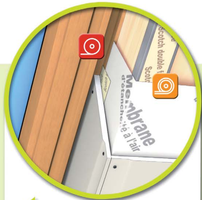
Raccordement à une fenêtre de toit
